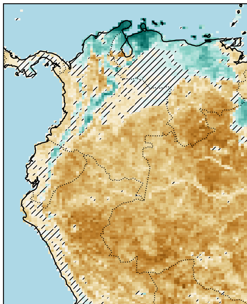
PCA ( p = 1.30\text{e-}01 )
